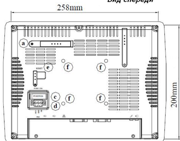
Вид сзади
