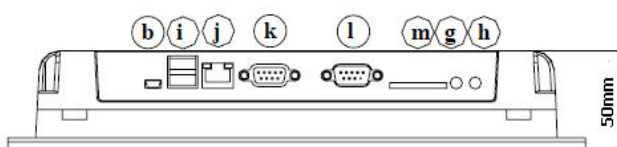
Вид снизу
