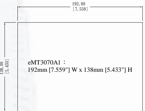
Cutout Dimensions
