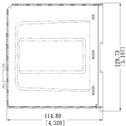
Вид сбоку
